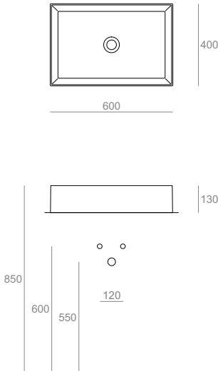
AG60 Lavabo 60 da appoggio Countertop washbasin 60 60.40.13
