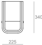
WASA07 Struttura d'appoggio per lavabo WA 07 Stand for washbasin WA 07 22,5.34.74
