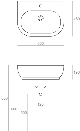
EL10 Lavabo 65 da appoggio o sospeso predisposto monoforo Countertop or wall-hung washbasin 65 pre-punched for single tap hole 65.48.19
