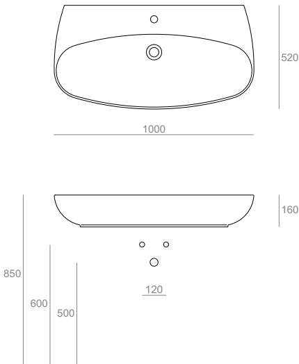
VI12 Consolle 100 da appoggio o sospesa monoforo Countertop or wall-hung console basin 100 for single tap hole 100.52.16
