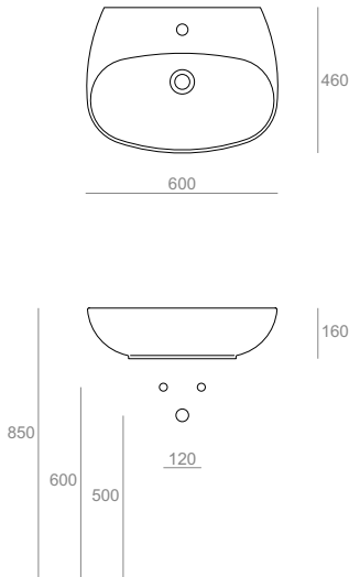
VI10 Lavabo 60 da appoggio o sospeso monoforo Countertop or wall-hung washbasin 60 for single tap hole 60.46.16
