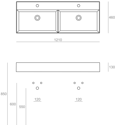
AG121D Lavabo 121 monoforo doppia vasca sospeso o da appoggio Wall-hung or countertop double bowl basin 121 121.46.13
