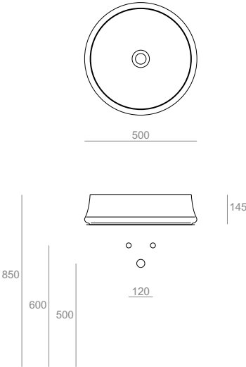
SH01 Lavabo Ø50 tondo da appoggio Round countertop washbasin Ø50 Ø50.114,5
