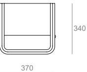
WASA08 Struttura d'appoggio per lavabo WA 08 Stand for washbasin WA 08 37.34.74
