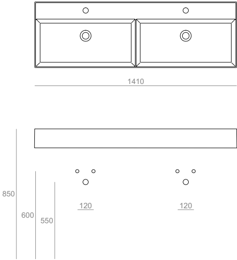
AG141D Lavabo 141 monoforo doppia vasca sospeso o da appoggio Wall-hung or countertop double bowl basin 141 141.46.13
