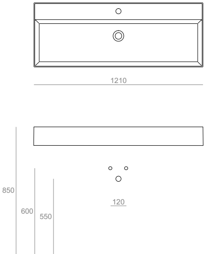
AG121 Lavabo 121 monoforo da appoggio o sospeso Countertop or wall-hung washbasin 121 for single tap hole 121.46.13
