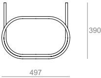
WASA02 Struttura d'appoggio per lavabo WA 02 Stand for washbasin WA 02 49,7.39.74
