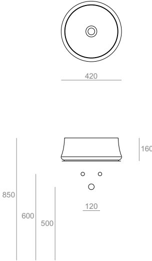
SH02 Lavabo Ø42 tondo da appoggio Round countertop washbasin Ø42 Ø42.16
