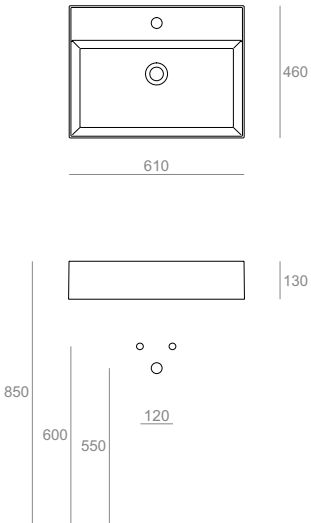
AG61 Lavabo 61 monoforo da appoggio o sospeso Countertop or wall-hung washbasin 61 for single tap hole 61.46.13
