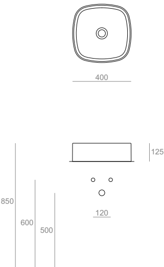
FO03 Lavabo 40 quadrato d'appoggio Square countertop washbasin 40 40.40.12,5
