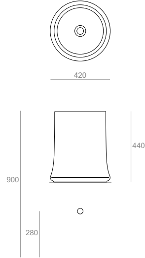
SH10 Lavabo Ø42 tondo da appoggio Round countertop washbasin Ø42 Ø42.44
