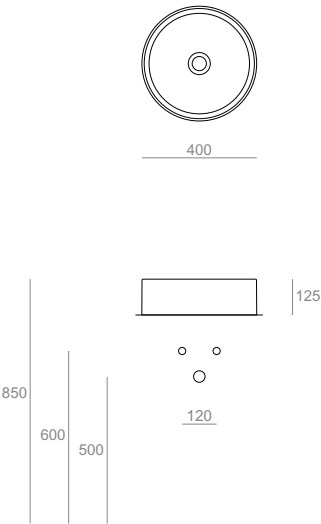
FO01 Lavabo Ø 40 tondo d'appoggio Round countertop washbasin Ø 40 Ø40.12,5
