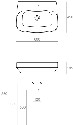
BB10 Lavabo 60 da appoggio o sospeso monoforo Countertop or wall-hung washbasin 60 for single tap hole 60.45.16
