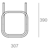
WASA03 Struttura d'appoggio per lavabo WA 03 Stand for washbasin WA 03 30,7.39.74
