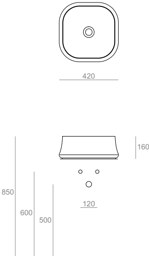
SH06 Lavabo 42 quadrato da appoggio Square countertop washbasin 42 42.42.16
