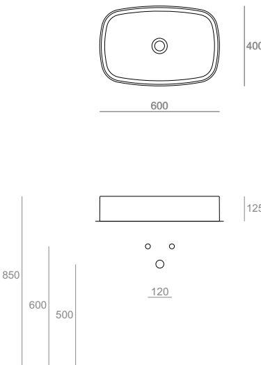
FO04 Lavabo 60 rettangolare d'appoggio Rectangular countertop washbasin 60 60.40.12,5
