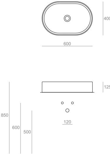
FO02 Lavabo 60 ovale d'appoggio Oval countertop washbasin 60 60.40.12,5
