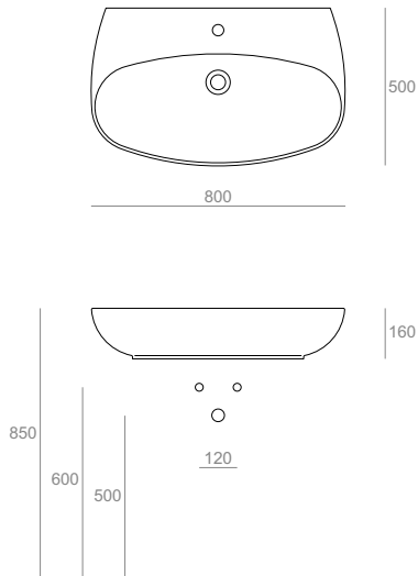
VI11 Lavabo 80 da appoggio o sospeso monoforo Countertop or wall-hung washbasin 80 for single tap hole 80.50.16
